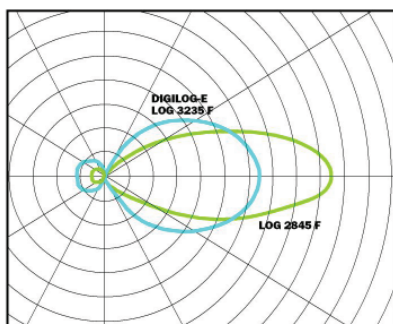
Diagramas de Radiación
