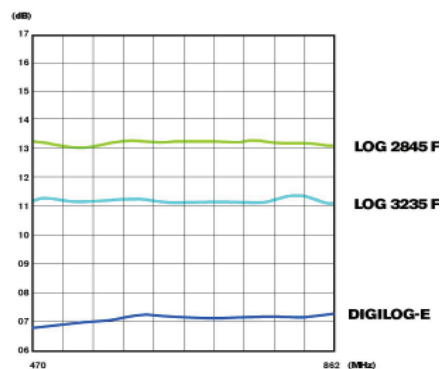
Diagramas de Ganancia (dB)
