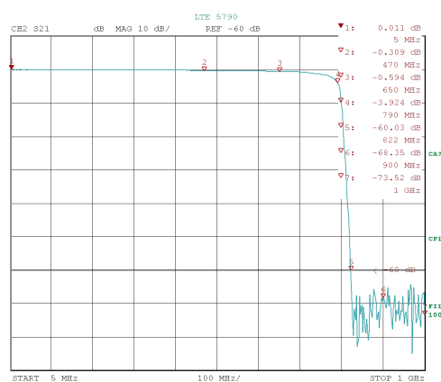
Gráfica de pérdidas de inserción Lte 5790
