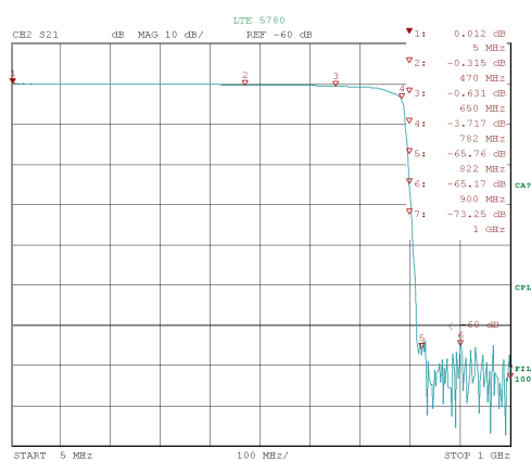
Gráfica de pérdidas de inserción Lte 5780
