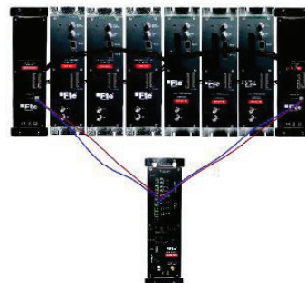
Redundancy 1:1
