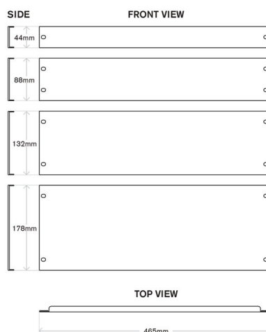
TP 1U - TP 2U - TP 3U - TP 4U dimensions
